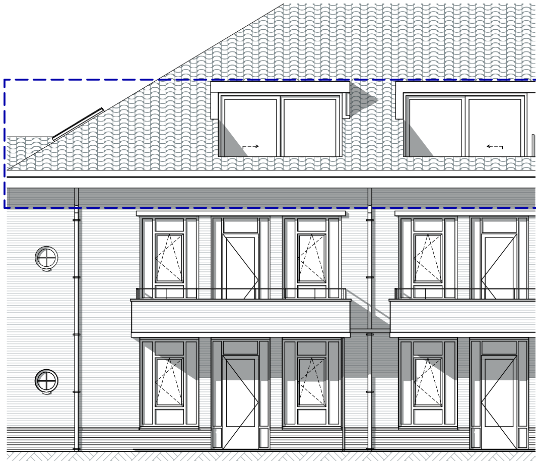
Oostgevel
