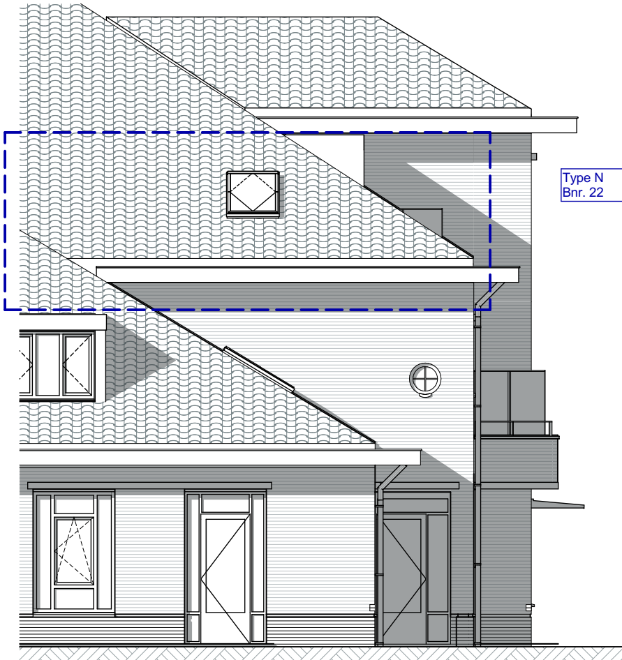
Zuidgevel
