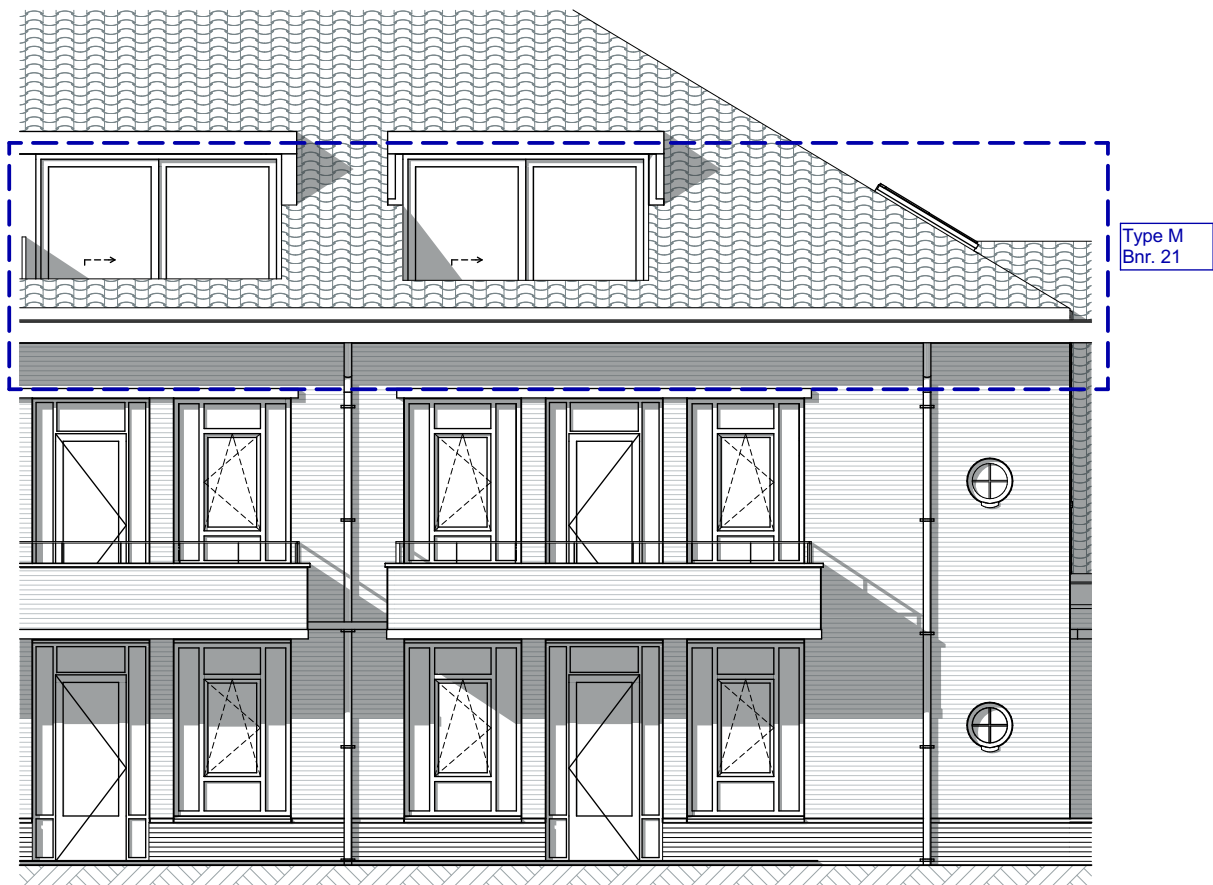
Westgevel
