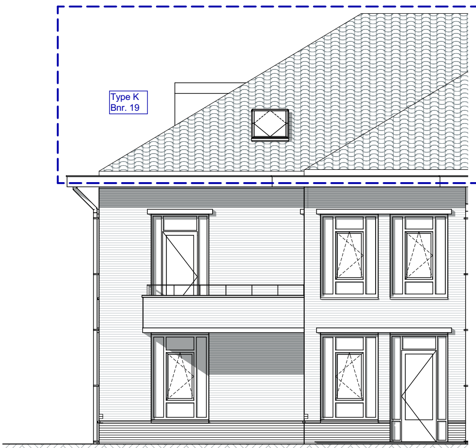
Westgevel
