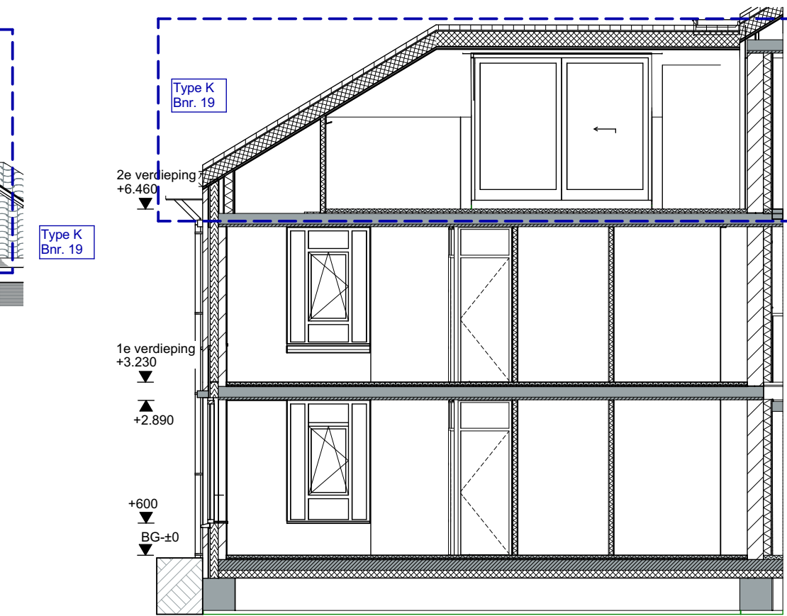
Doorsnede Type K
