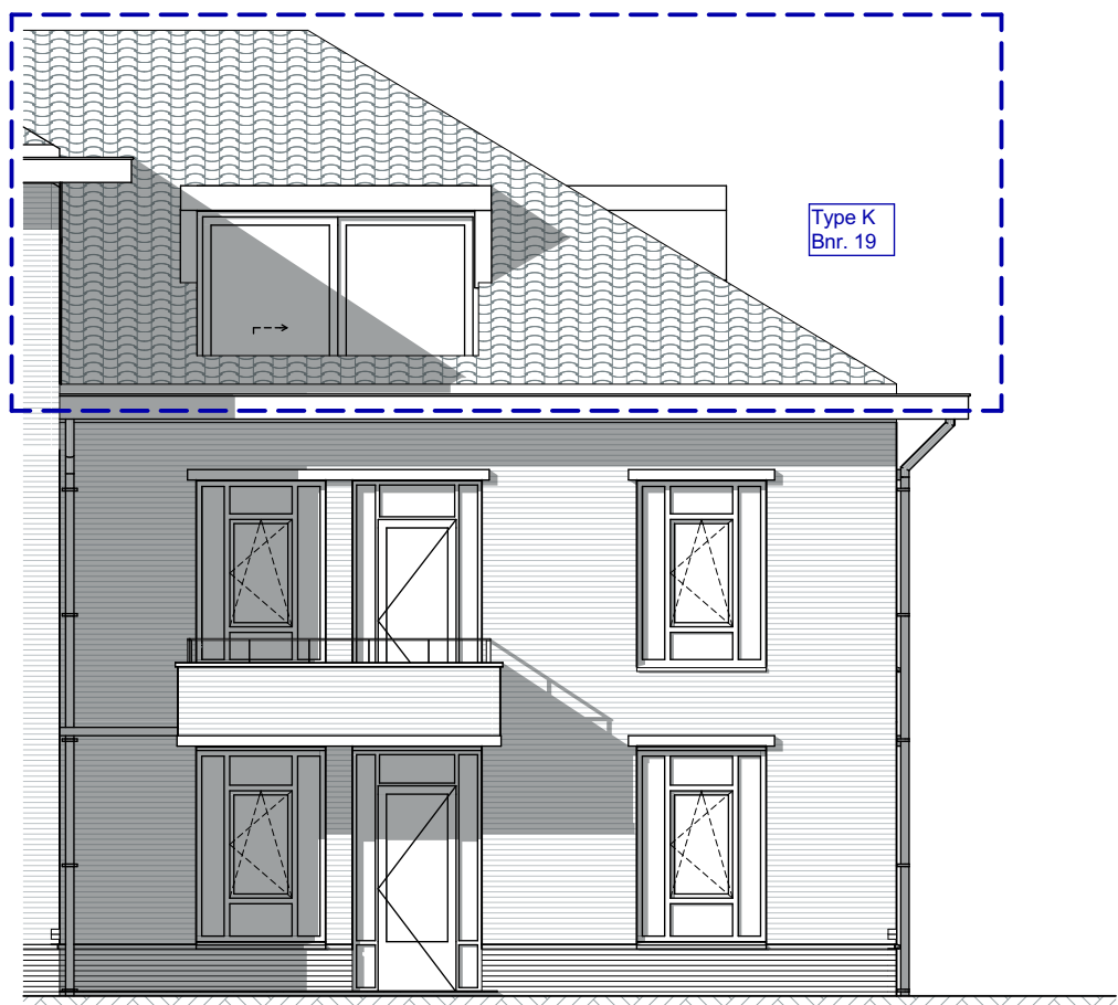
Oostgevel
