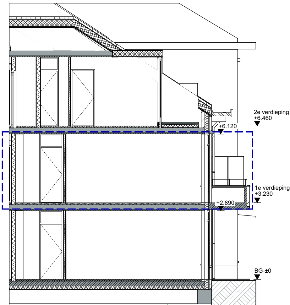
Doorsnede Type H
