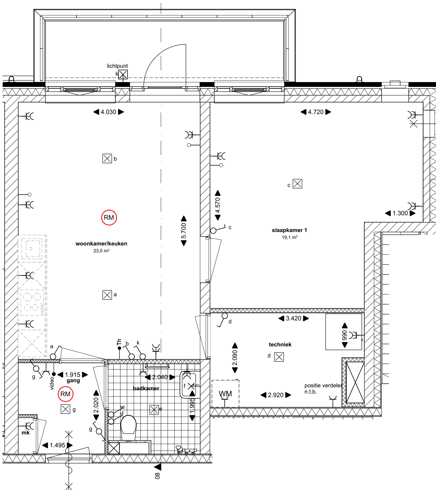
1e verdieping Type H Bouwnummer 16
