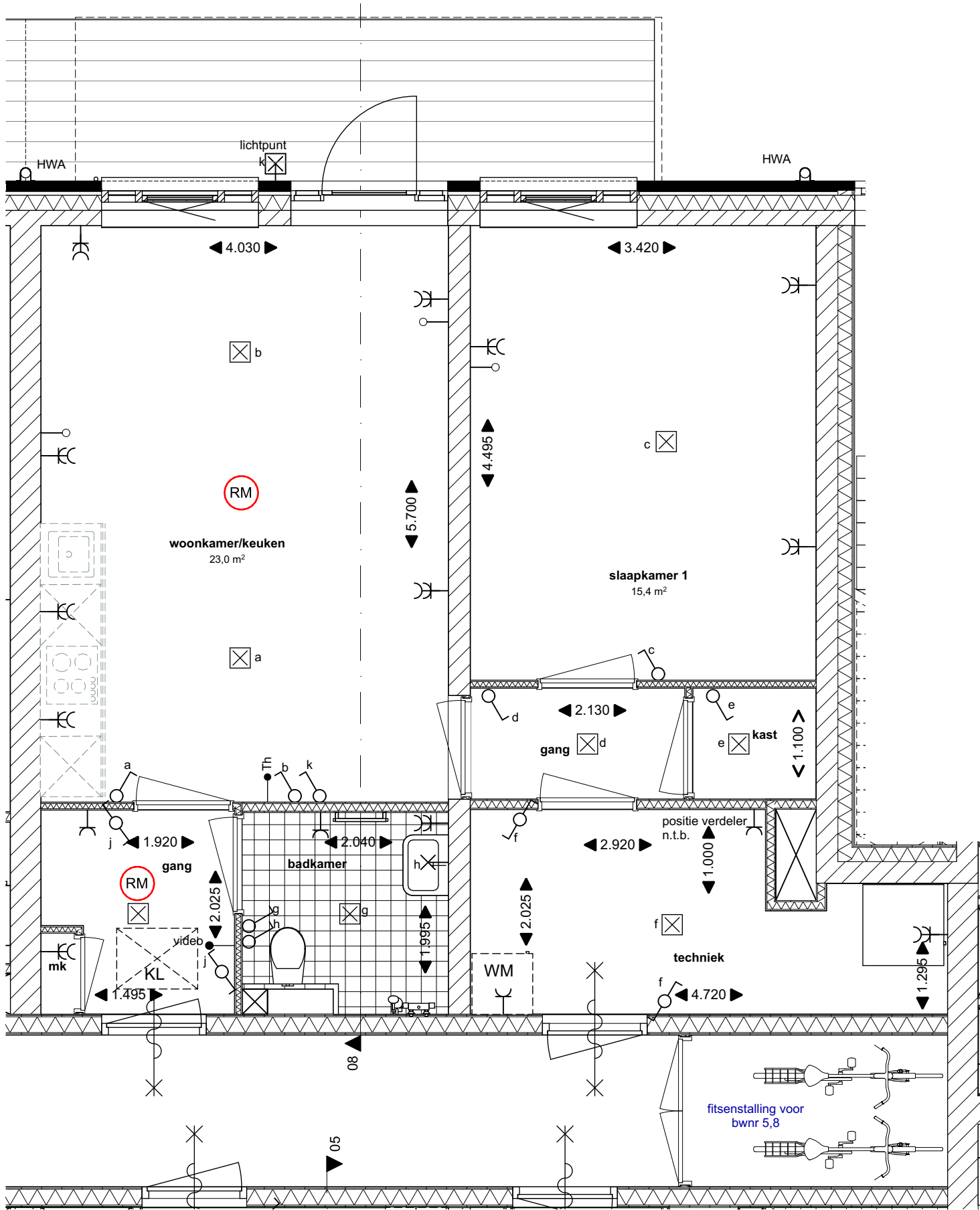
Begane grond Type F Bouwnummer 8
