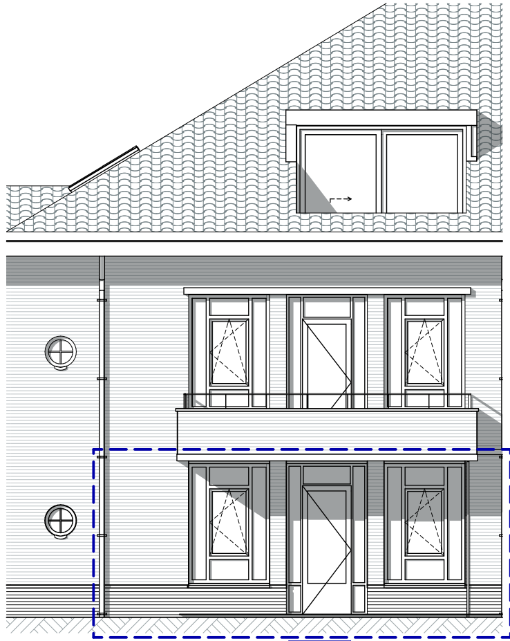
Oostgevel
