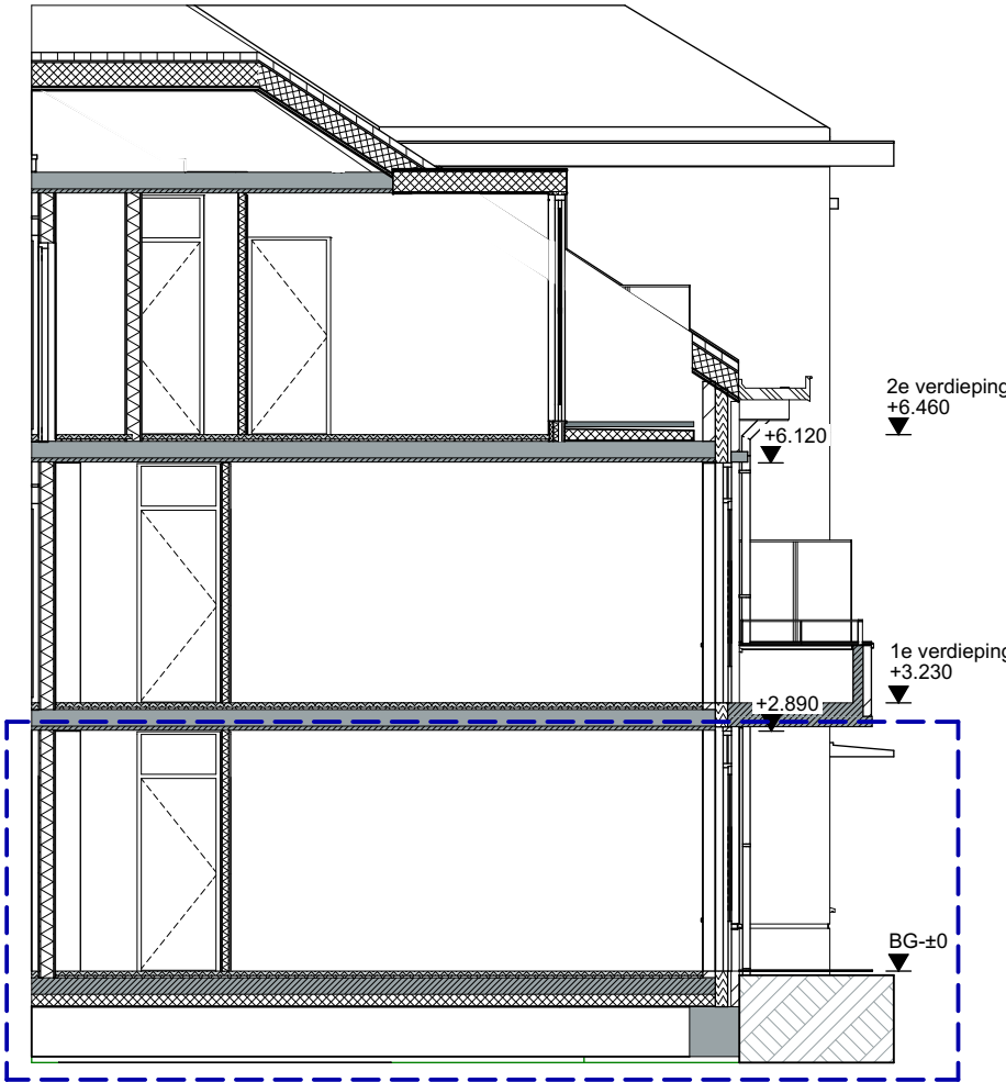
Doorsnede Type F
