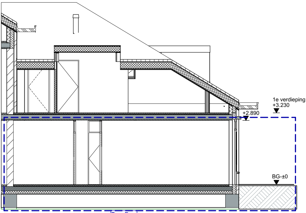
Doorsnede Type E
