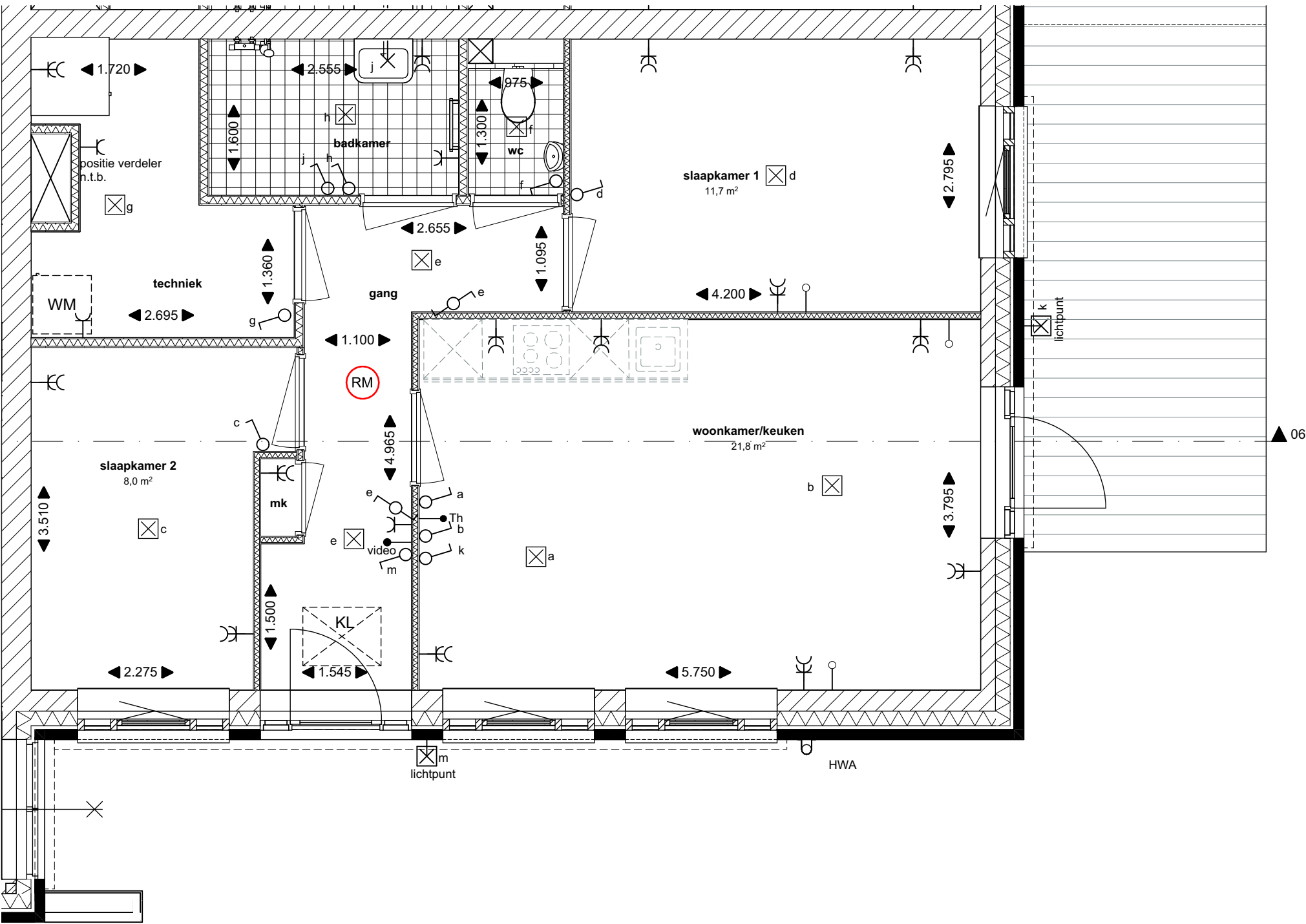
Begane grond Type E Bouwnummer 6
