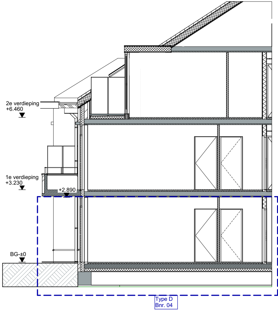
Doorsnede Type D
