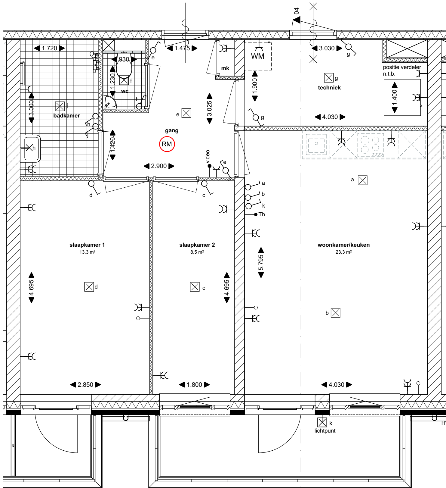
1e verdieping Type D
