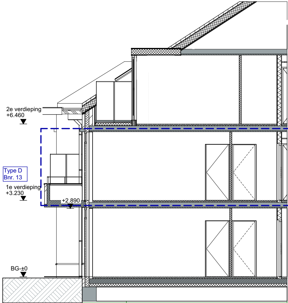
Doorsnede Type D
