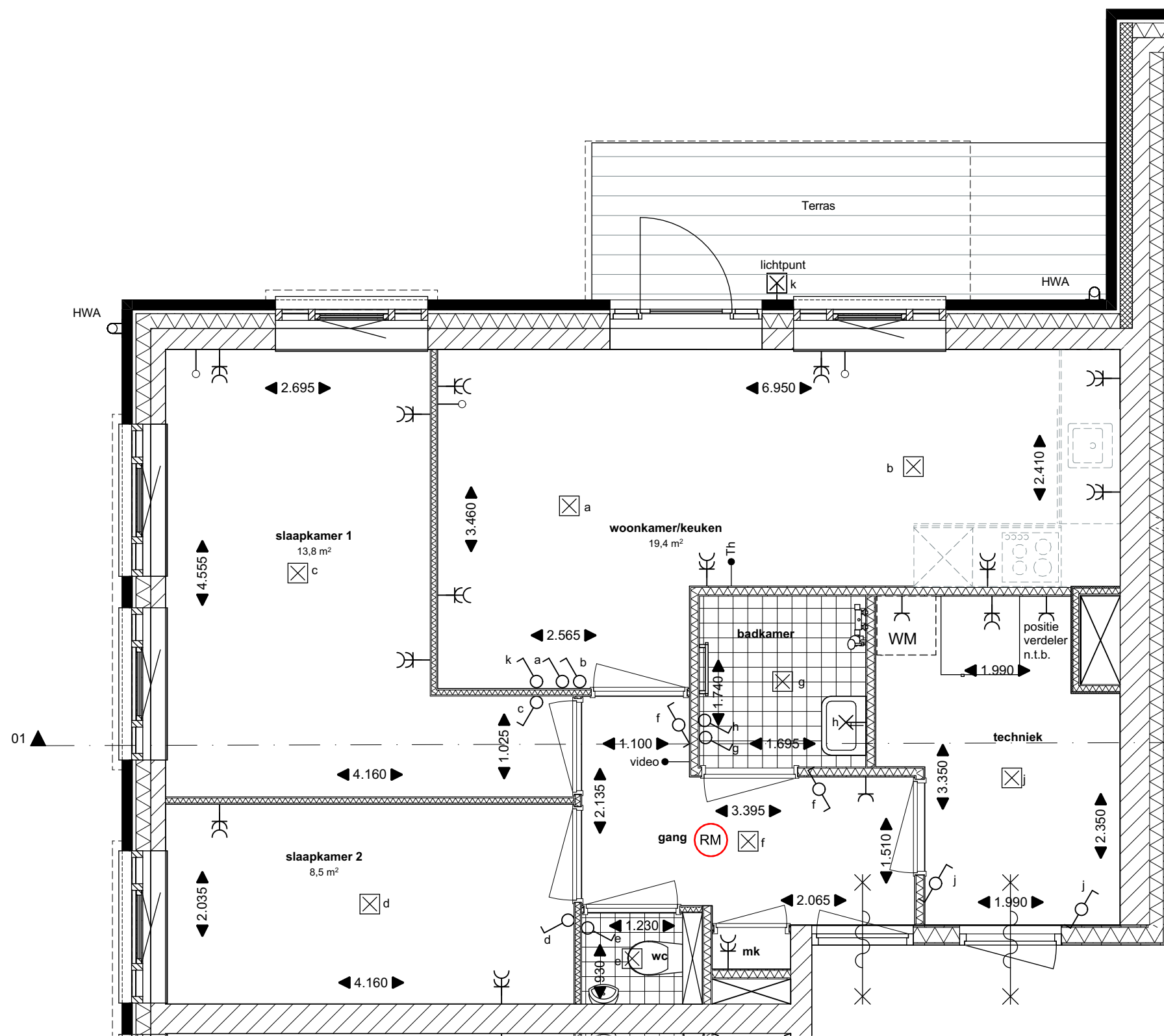
Begane grond Type A Bouwnummer:1
