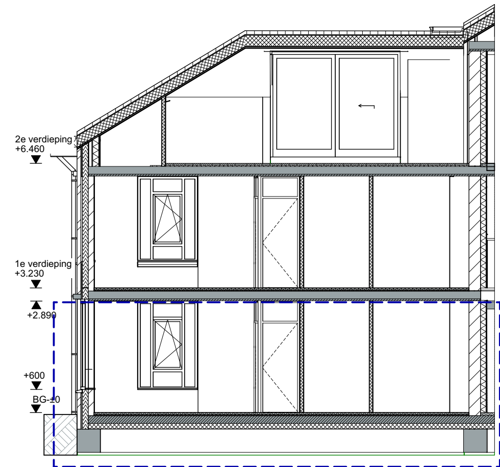
Doorsnede Type A
