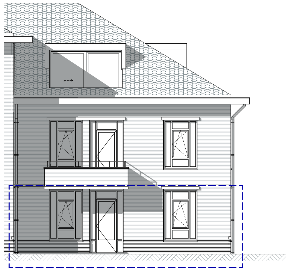
Oostgevel
