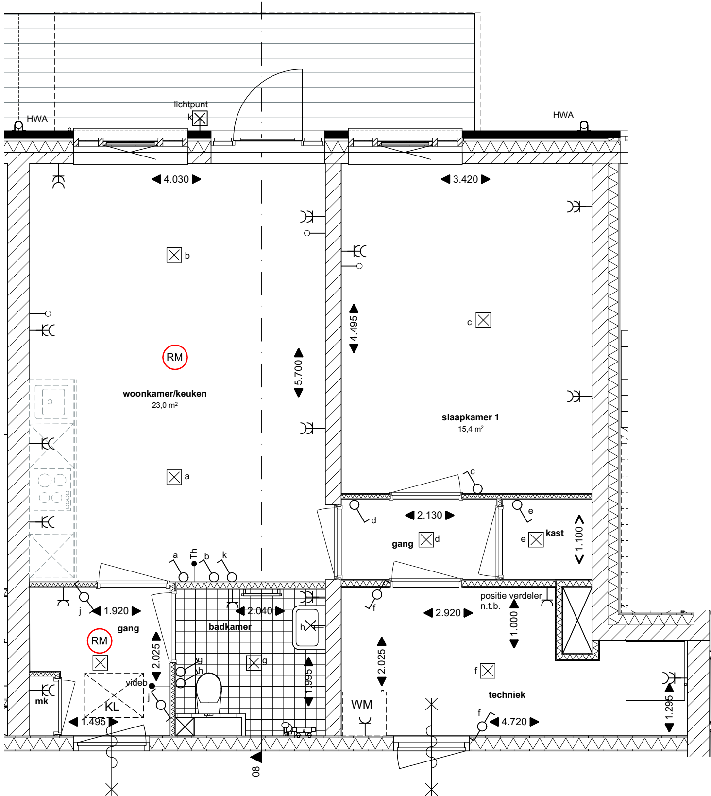
Begane grond Type F Bouwnummer 8
