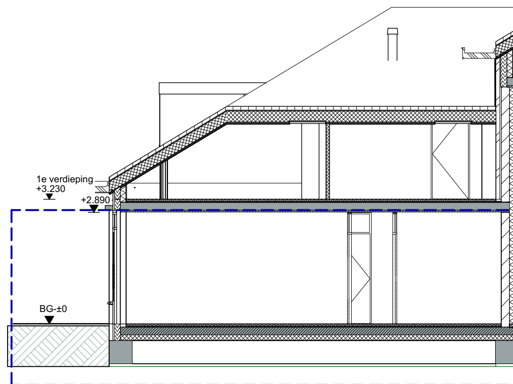
Doorsnede Type Esp
