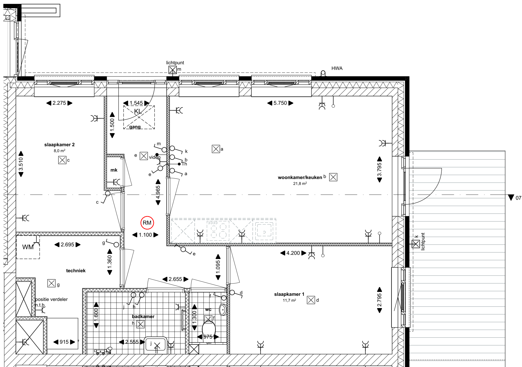
Begane grond Type Esp Bouwnummer 7
