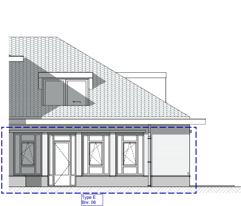
Oostgevel
