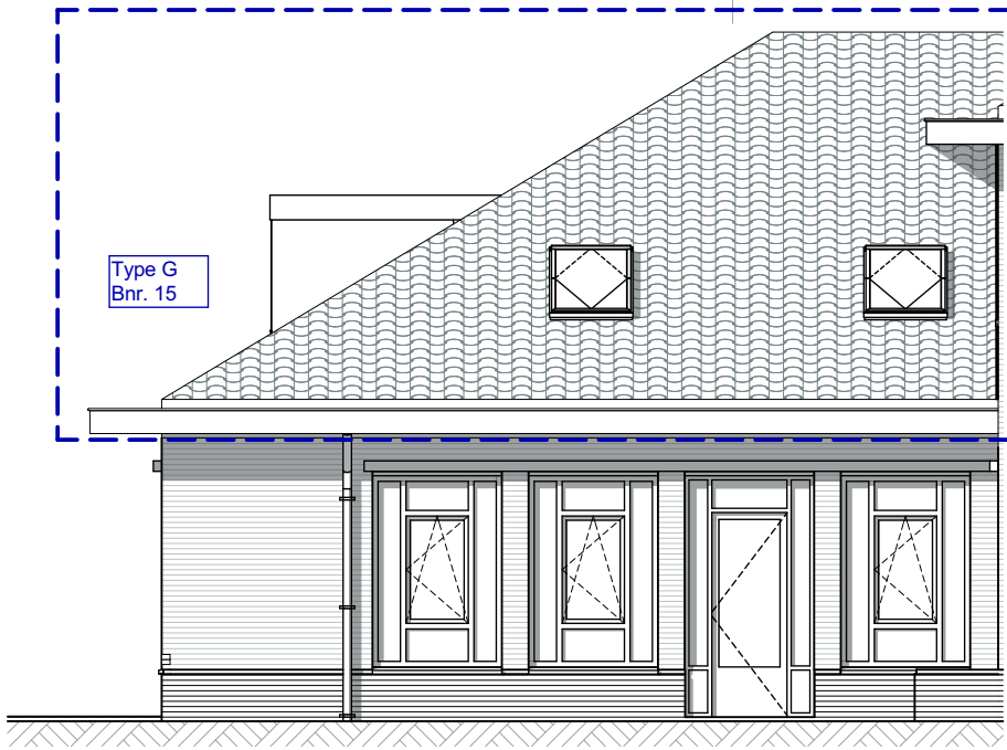
Westgevel
