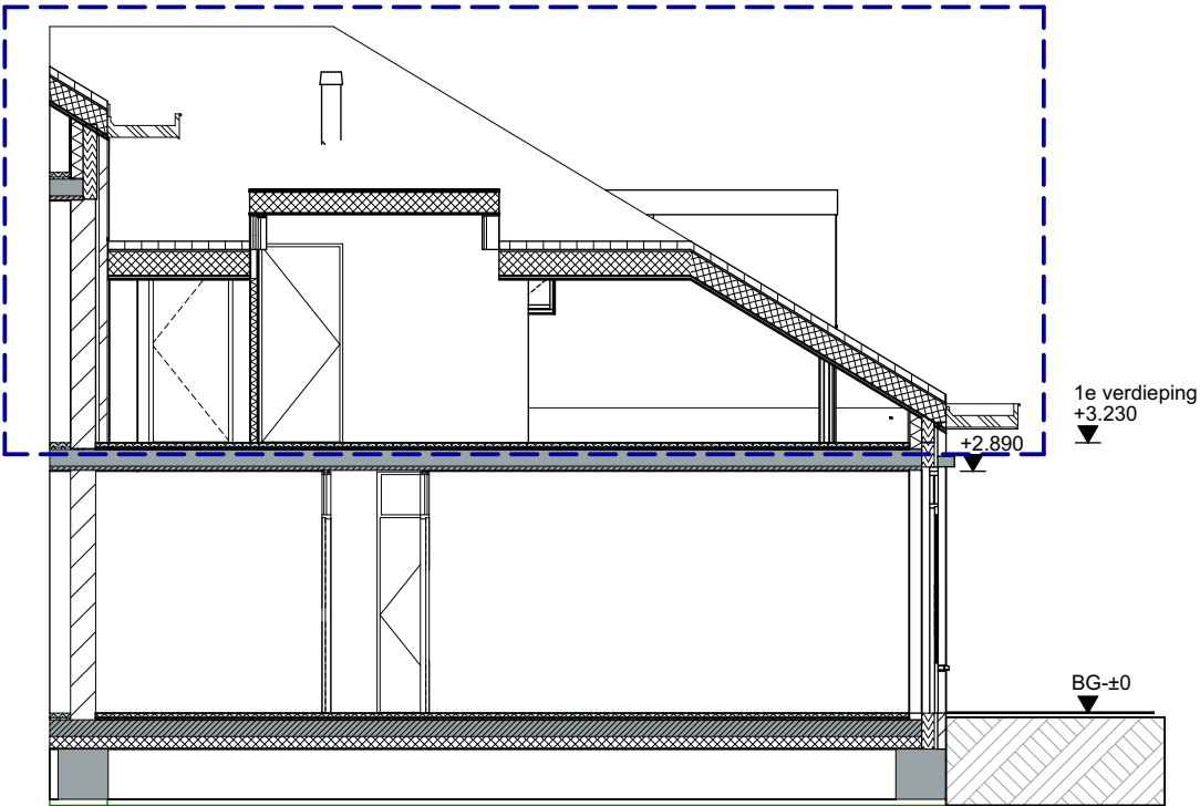
Doorsnede Type G
