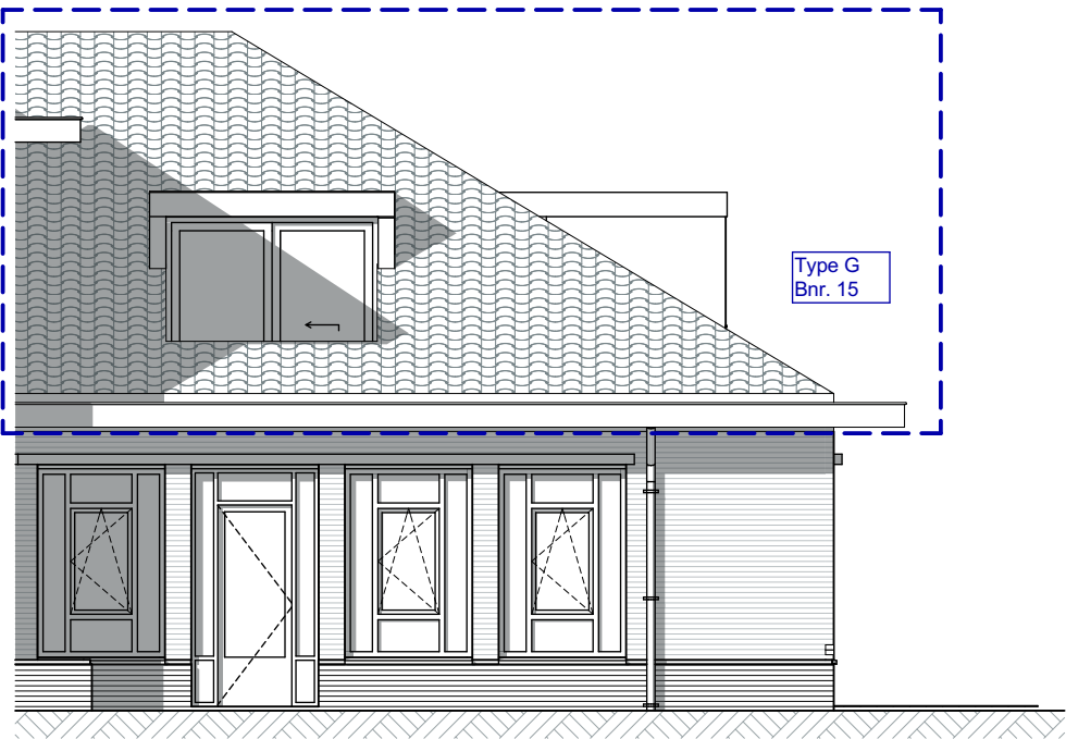
Oostgevel
