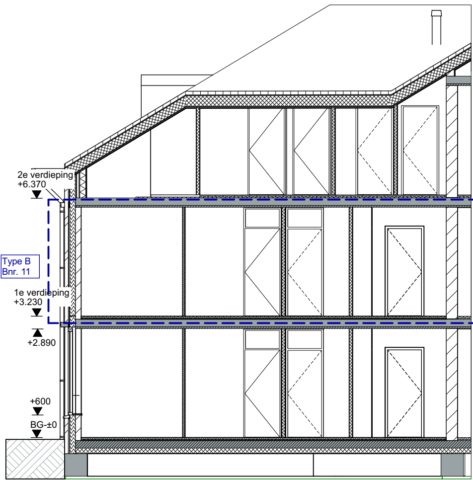
Doorsnede Type B
