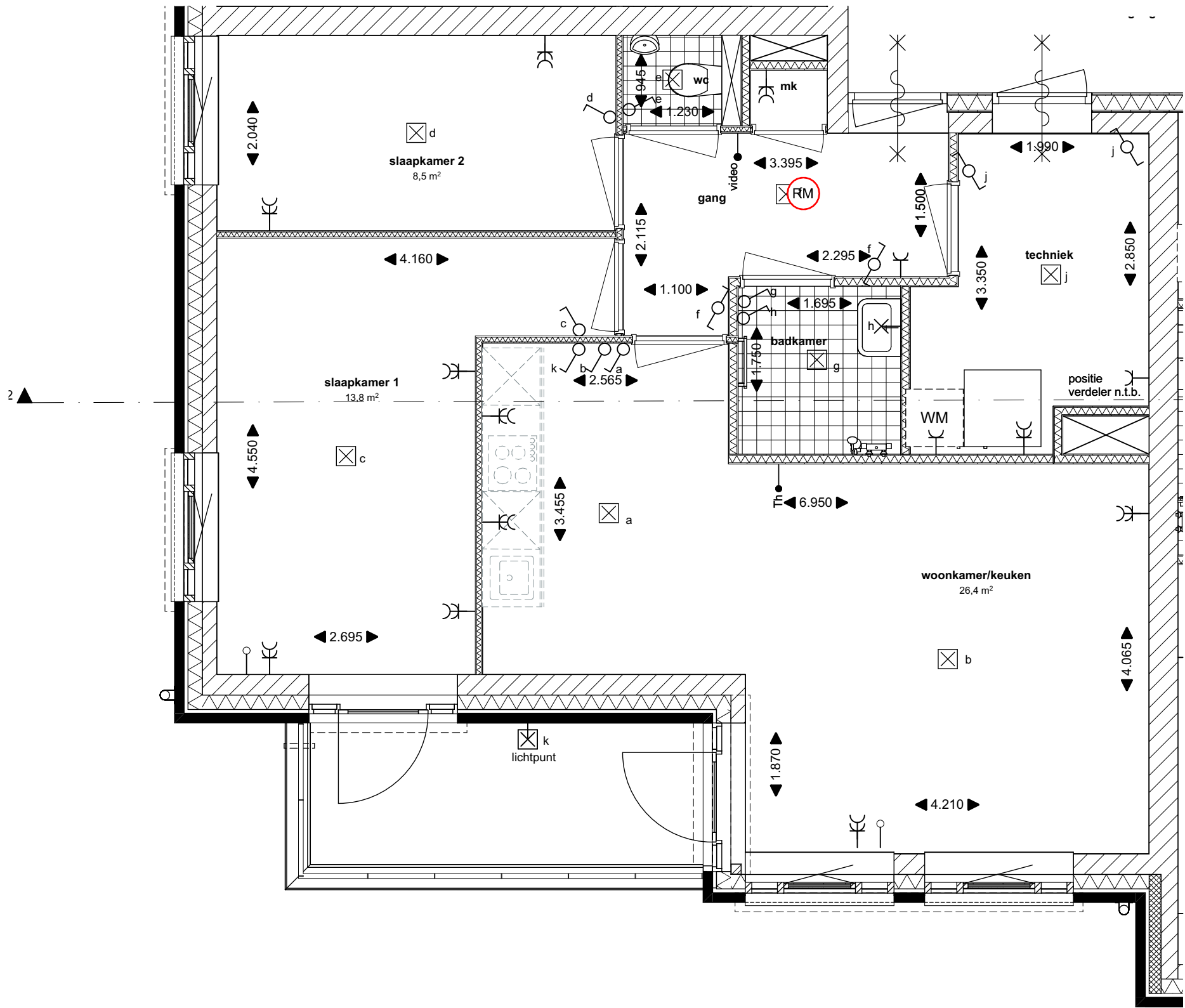
1e verdieping Type B
